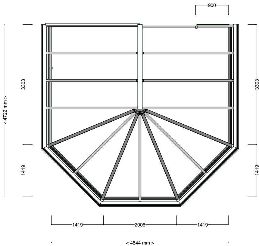
Widok z góry wymiarowany
